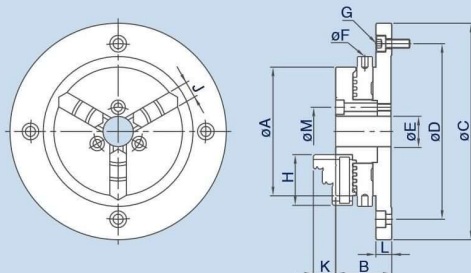
尺寸圖 » Dimensions
