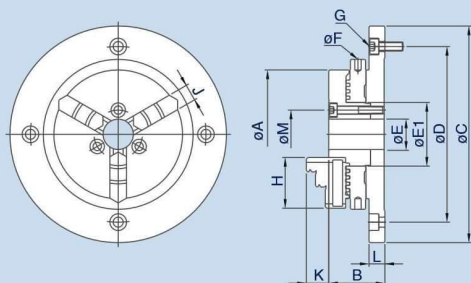
尺寸圖 » Dimensions
