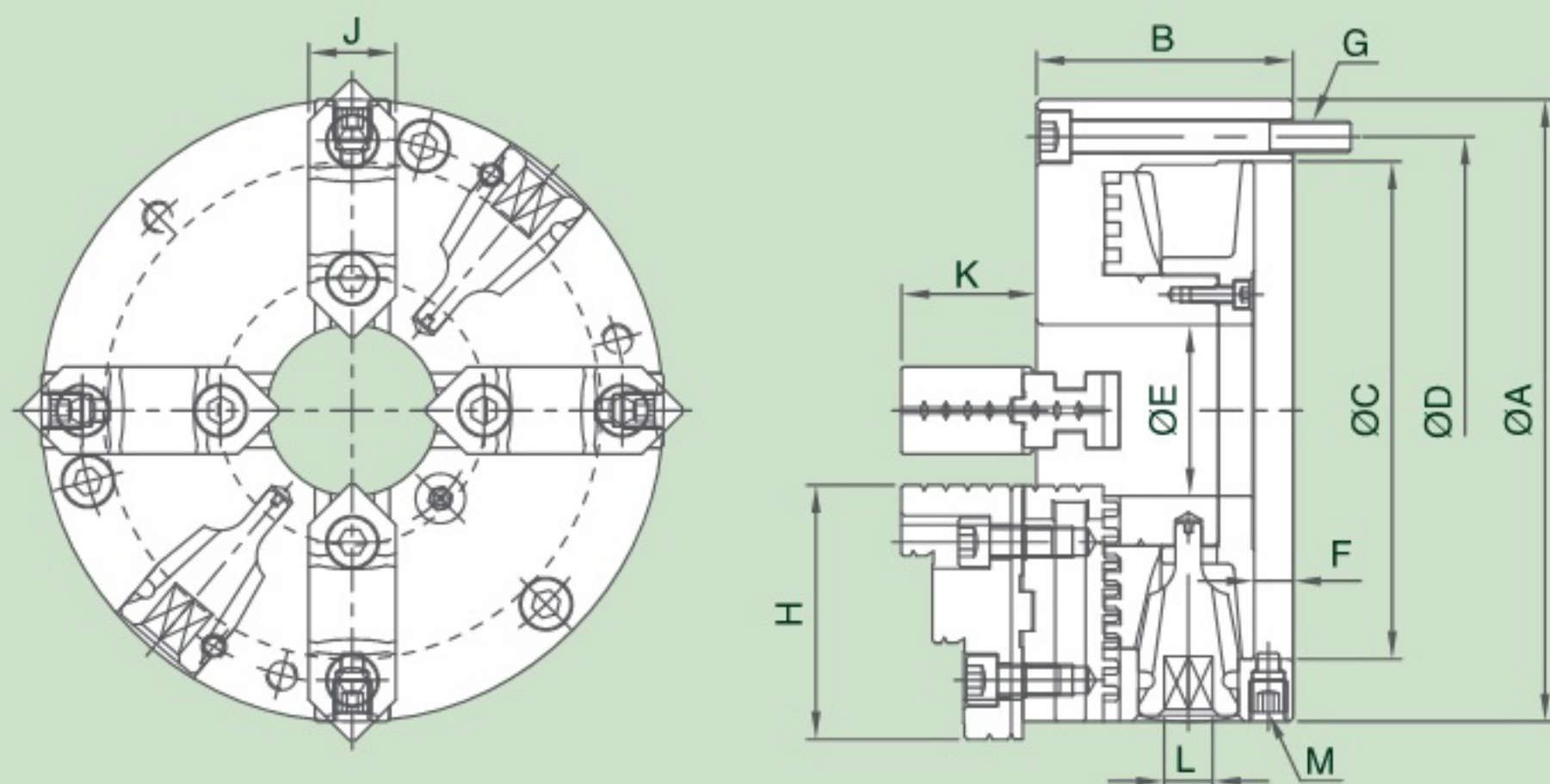
尺寸圖 » Dimensions
